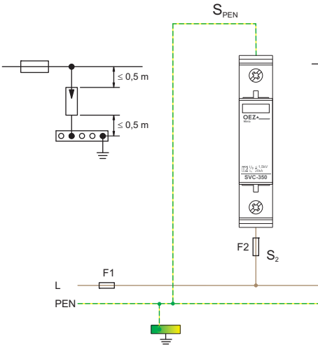
TN-C
